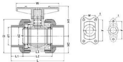
Кран шаровой промышленного применения, муфтовые окончания, EPDM, IPS d75
