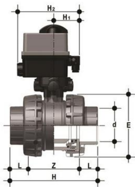
Шаровой кран VXE ПВХ с пневмоприводом НЗ, муфтовые окончания, FKM, FIP d110 (DN90)
