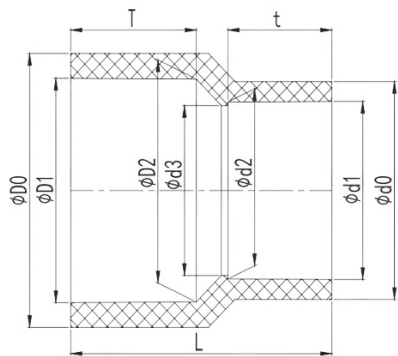
Муфта редукционная ПВХ IPS 400х315
