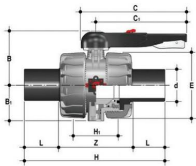
Шаровой кран промышленного применения VKD с патрубками из ПЭ (CVDE) (уплотнение FKM) PP-H d90
