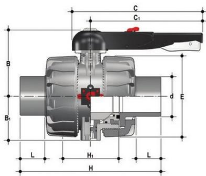
Шаровой кран промышленного применения VKD C втулочными окончаниями (уплотнение EPDM) PP-H d75 (DN65)
