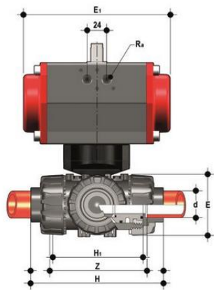
3-х ходовой шаровой кран ТКД с пневмоприводом ДвД с муфтовыми окончаниями, Т-шар (уплотнение FKM) PP-H d16 (DN10)
