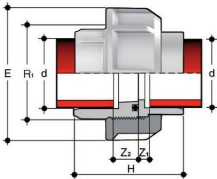
Муфта разборная ПВДФ d40 SDR21 PN16
