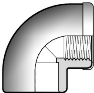
Отвод 90° переходной на ВР с кольцом ПВХ FIP 32x1
