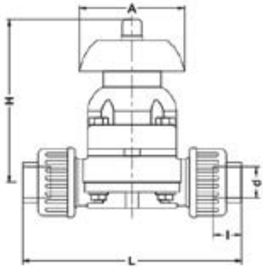
Мембранный клапан IDK ПВХ с муфтовыми окончаниями, PTFE, IPS d110 (DN100)
