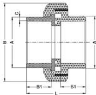
Муфта разборная для стыковой сварки PP-H IPS d20 PN 10
