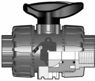
Шаровой кран промышленного применения VKD ХПВХ с резьбовыми окончаниями R2" (DN50)
