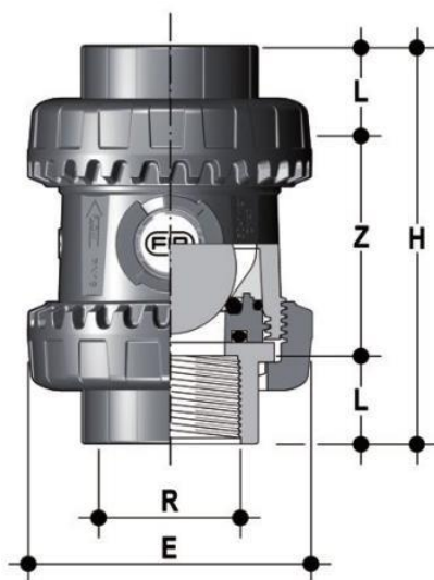
Шаровой обратный клапан SXEFV ПВХ; с резьбовыми окончаниям, FKM, FIP R2" (DN50)
