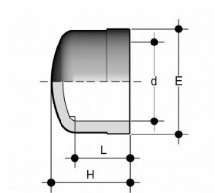
Заглушка клеевая ПВХ FIP d90
