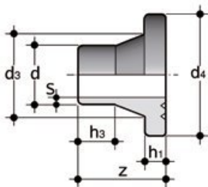
Бурт под фланец для стыковой сварки PP-H FIP (PN6) d800 SDR17.6 PN6
