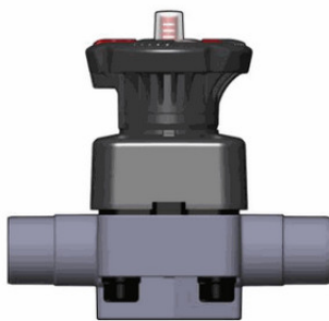
Мембранный клапан DK с втулочными окончаниями (уплотнение EPDM / мембрана EPDM) PP-H d63 (DN50)
