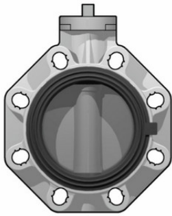
Дисковый затвор промышленного применения FКОAMFM со свободным штоком (уплотнение FKM) PP-H d315 (DN300)
