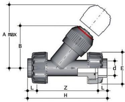
Угловой обратный клапан VRUIV ПВХ с разборными муфтовыми окончаниями, FKM, FIP d16 (DN10)
