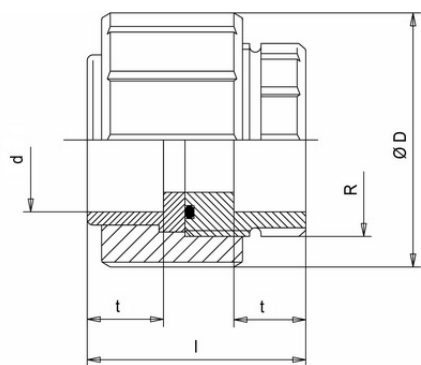
Муфта разборная ПВДФ (Simona) d63 SDR21 PN16
