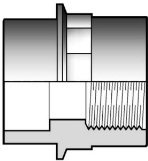
Двойной муфтовый адаптер с ВР ПВХ FIP 32x25x3/4
