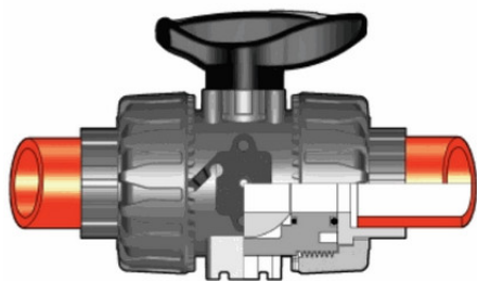
Шаровой кран промышленного применения VKD с муфтовыми окончаниями (уплотнение FKM) PP-H d63
