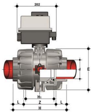
Шаровой кран VKD с эл.приводом 24V AC/DC, муфтовые окончания, DN65-100 (уплотнение FKM) PP-H d90 (DN80)
