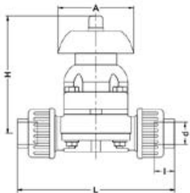
Мембранный клапан IDK ПВДФ с муфтовыми окончаниями d110(DN100)
