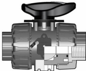
Шаровой кран для регулирования потока VKRFM с резьбовыми окончаниями (уплотнение EPDM) PP-H 1"
