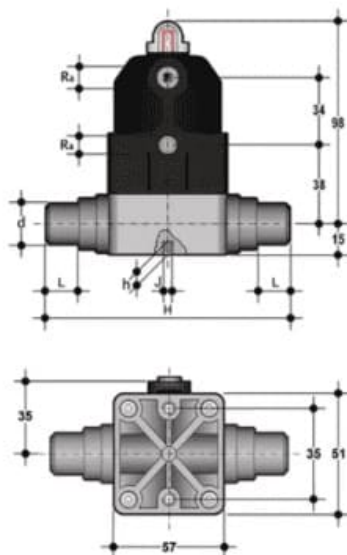
Компактный мембранный клапан CM с пневмоприводом НО с резьбовыми окончаниями (уплотнение EPDM/мембрана EPDM) PP-H R3/8" (DN12)
