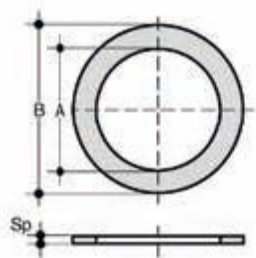
Плоское уплотнение IPS под фланцевое соединение (EPDM) d50
