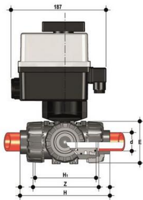
3-х ходовой шаровой кран TKD с эл.приводом 24V AC/DC, муфтовые окончания, L-шар (уплотнение EPDM) PP-H d25 (DN20)
