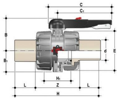
Шаровой кран промышленного применения VKD с патрубками (CVDM) (уплотнение FKM) PP-H d110 (DN100)
