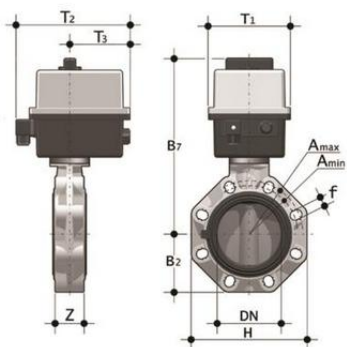
Дисковый затвор промышленного применения FK ПВХ с эл.приводом 90-240V, EPDM, FIP d10" (DN250)
