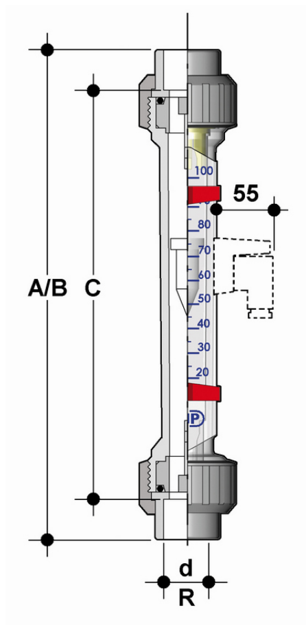
FS ротаметр для воды; корпус: полисульфон; поплавок с магнитом d75
