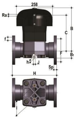
Мембранный клапан VM ПВДФ с пневмоприводом НО, PN10 с фланцевыми окончаниями d110 (DN90)
