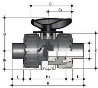
Шаровый кран ПВХ для регулирования потока VKR со втулочными окончаниями, EPDM, FIP d50 (DN40)
