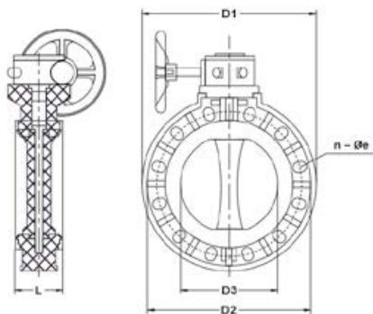
Затвор дисковый ПВХ с редуктором промышленный IPS (Model B) 16" (DN400)
