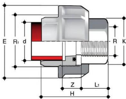
Муфта переходная разборная ВР ПВДФ 40х1 1/4 SDR21 PN16
