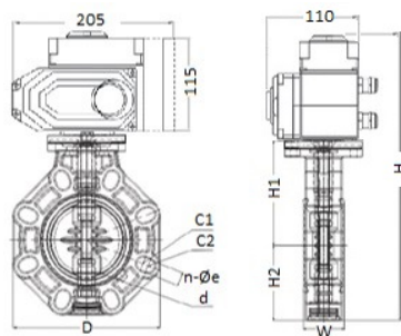
Дисковый затвор IFK ПВДФ с электрическим приводом 220V AC, EPDM, IPS d110 (DN100)
