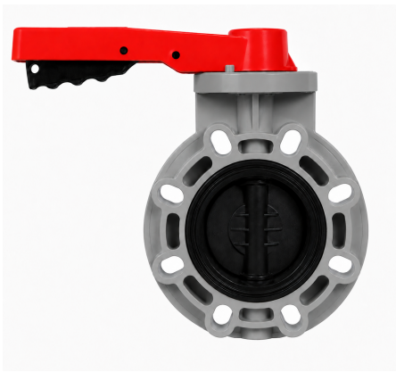
Затвор дисковый в корпусе FRPP (диск - НПВХ) с рукояткой промышленного применения EPDM IPS 90 (DN80)
