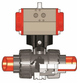
Шаровой кран VKD с пневмоприводом ДвД с муфтовыми окончаниями (уплотнение EPDM) PP-H d50 (DN40)
