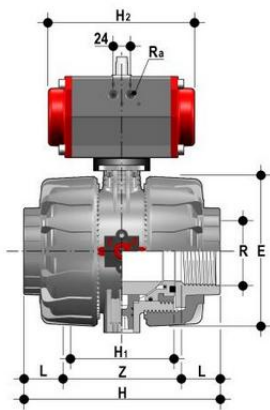
Шаровой кран VKD ПВХ с пневмоприводом НЗ с резьбовыми окончаниями, EPDM, FIP R3" (DN80)
