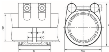
Соединительная муфта GRIP Ø54.0-168.3, EPDM, W5 d70
