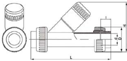
Фильтр сетчатый ХПВХ IPS d90
