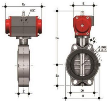
Дисковый затвор общего применения FE ПВХ с пневмоприводом НЗ, EPDM, FIP d110 (DN100)
