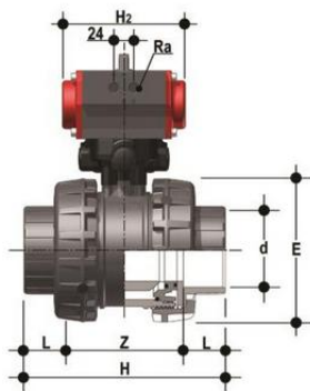
Шаровой кран общего применения VXE ХПВХ с пневмоприводом НЗ с муфтовыми окончаниями d110 (DN90)
