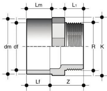
Двойной муфтовый адаптер с НР ПВХ FIP 75x63x2
