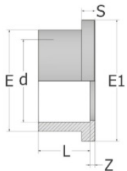
Бурт ХПВХ Comer d160 PN16
