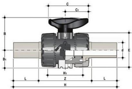
Шаровой кран VKD ПВДФ с длинными патрубками d50 (DN40)
