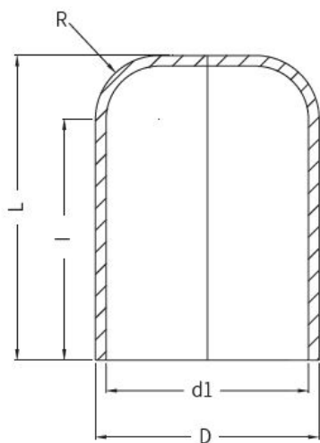
Заглушка ПВДФ для стыковой сварки d25 PN 16
