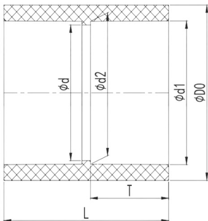
Муфта соединительная ПВХ IPS d400
