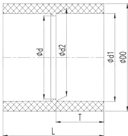
Муфта соединительная ПВХ IPS d225
