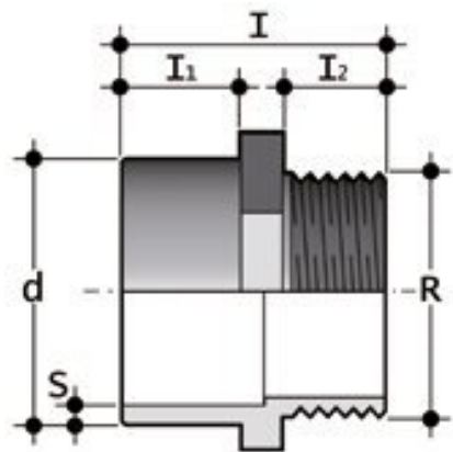
Адаптер с наружной резьбой PP-H FIP 63x2 SDR11 PN6
