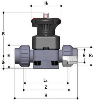
Мембранный клапан ДК ХПВХ с разборными резьбовыми окончаниями R2" (DN50)
