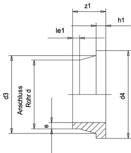
Бурт ПВДФ (Simona) d200 SDR33 PN10
